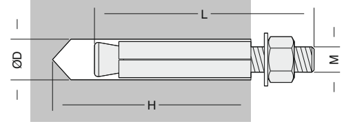
EAE Çekmeli Boru Tipi Dübel
