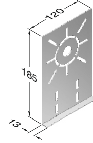
Tek Taraflı Kanal Birleştirme Contası
